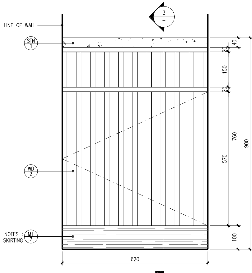
CASHIER COUNTER - ELEV. 2 1 : 10 0 10 20 Cm
