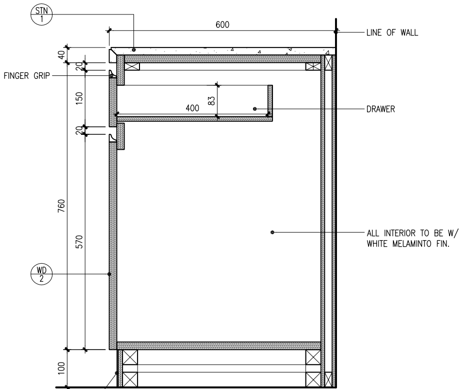
CASHIER COUNTER - SECT. 3 1 : 10 0 10 20 Cm
