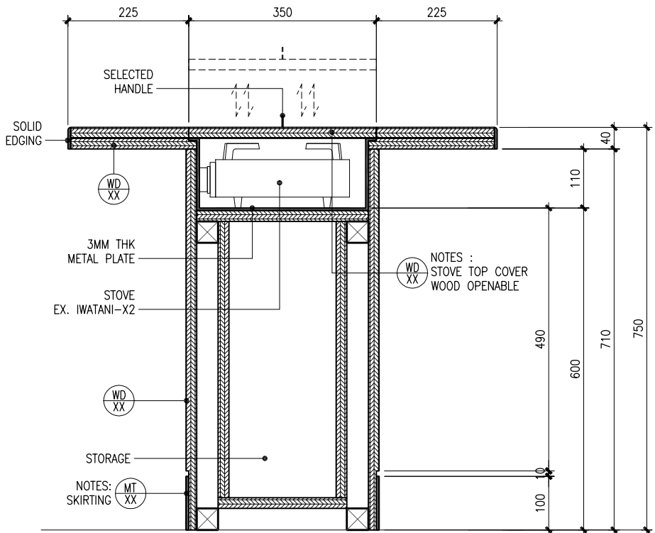
BOOTH TABLE - SECT 3 1 : 10 0 10 20 Cm
