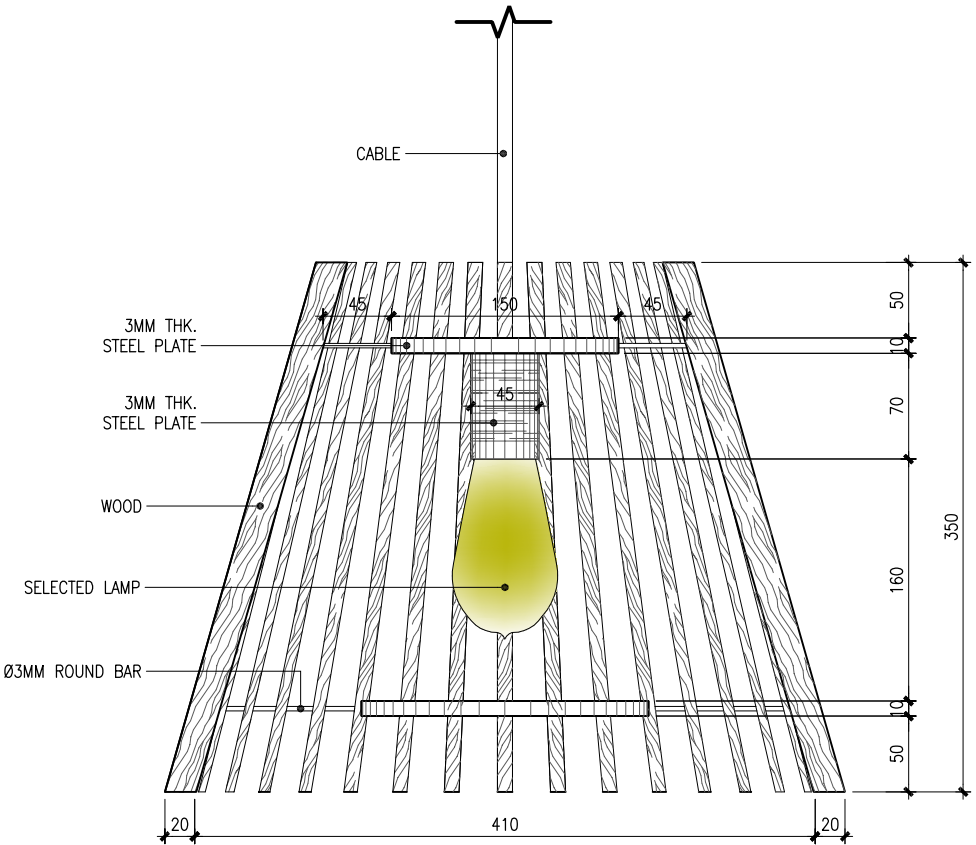
PENDANT LAMP - SECT 3
