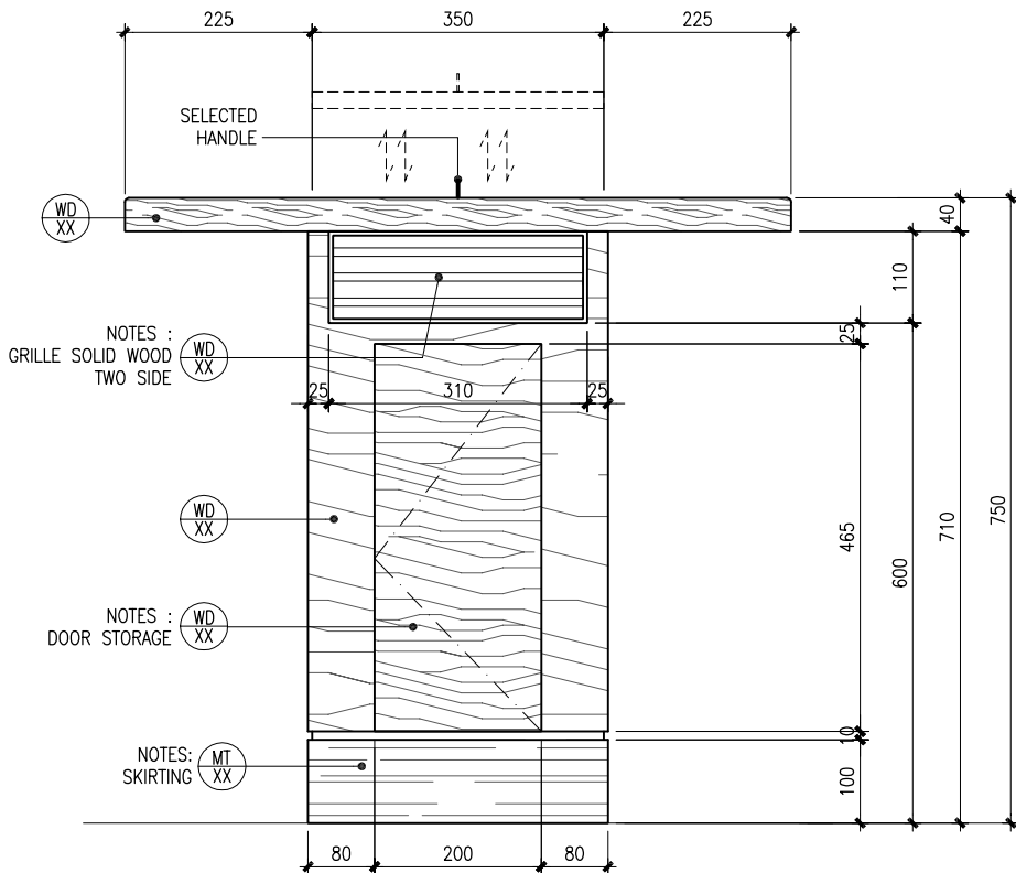
BOOTH TABLE - ELEV 1 1 : 10 0 10 20 Cm
