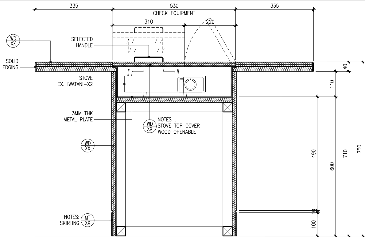
BOOTH TABLE - SECT 2 1 : 10 0 10 20 Cm
