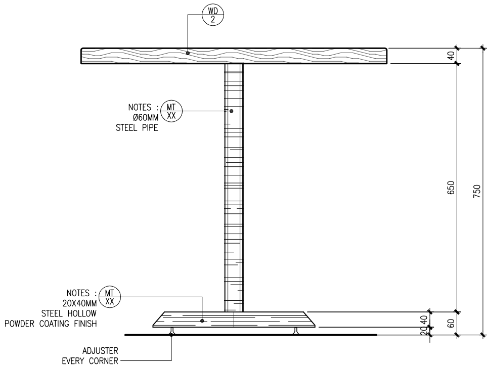
DINING TABLE - ELEV 2
