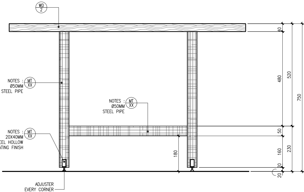
DINING TABLE - ELEV 2
