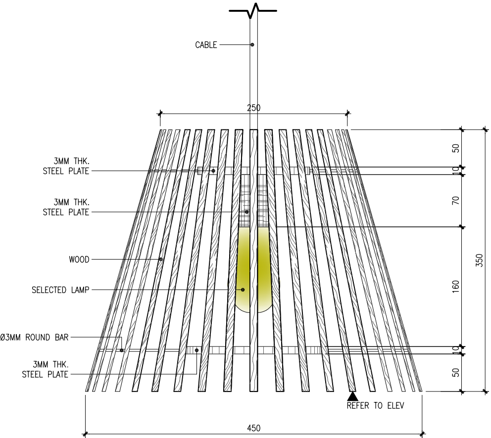
PENDANT LAMP - ELEV 2
