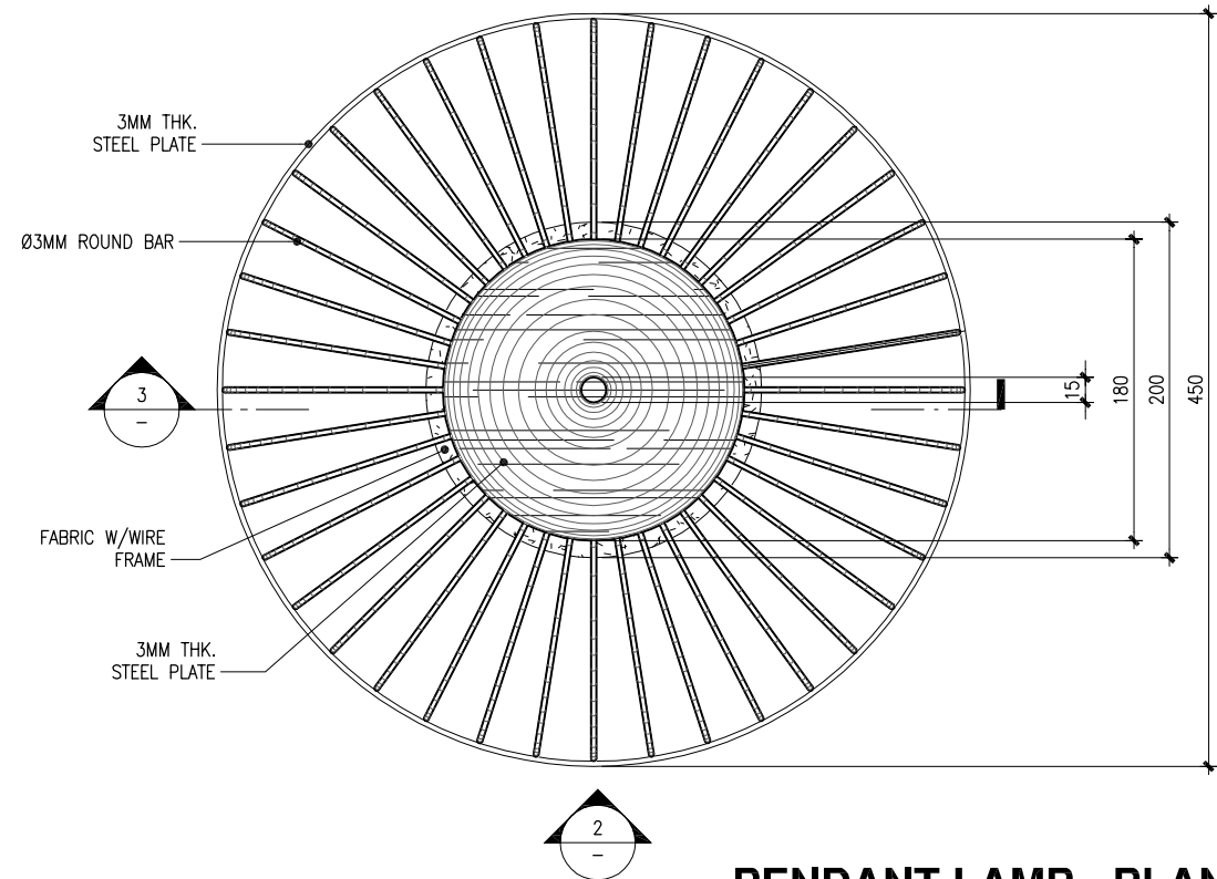
PENDANT LAMP - PLAN 1
