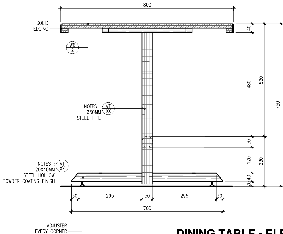
DINING TABLE - ELEV 3
