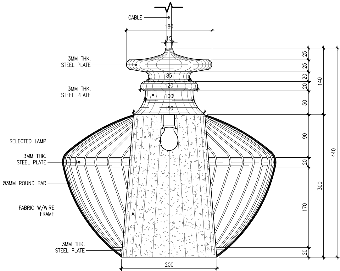
PENDANT LAMP - SECT 3
