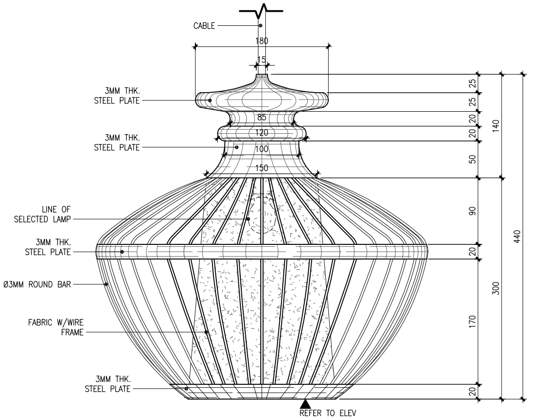
PENDANT LAMP - ELEV 2
